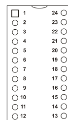
Ansicht von oben/ Top view
