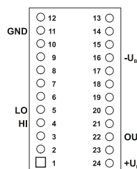
Ansicht von unten/ Bottom view
