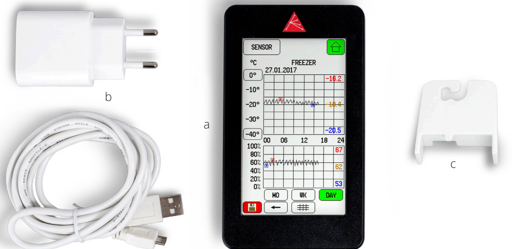
Aranet MINI kit: a) Aranet MINI gateway; b) AC power adapter with USB cable; c) Gateway stand.
